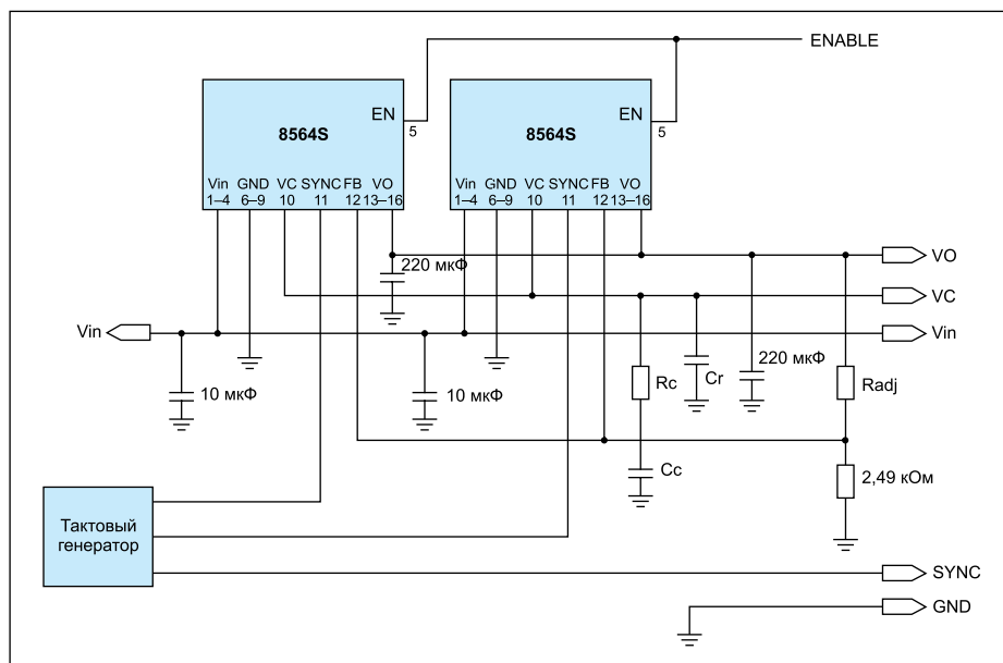
Рис. 4. Параллельное соединение двух модулей MHP8564S
