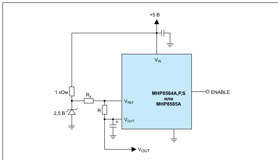
Рис. 3. Схема подключения MHP8564A для получения выходного напряжения менее 1,21 В
