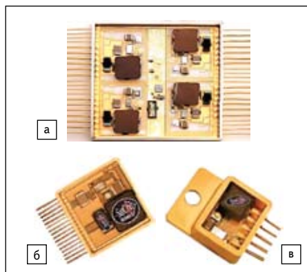
Рис. 1. Внешний вид радиационно-стойких POL-преобразователей: а) MHP8566; б) MHP8564; в) MHP8565
