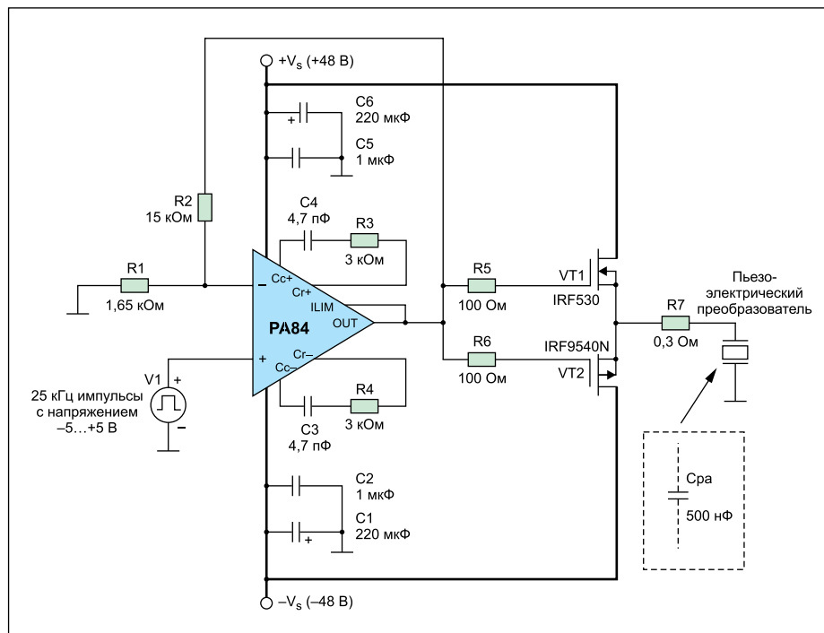
Рис. 4. Типовая схема подключения ОУ PA84
