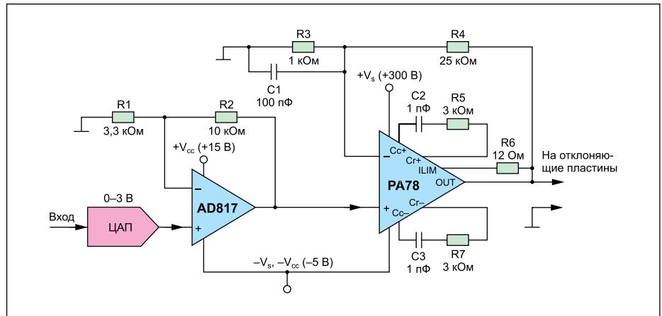
Рис. 7. Схема управления отклоняющимися пластинами
