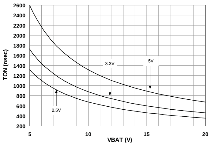
TON vs. VBAT - V_{OUT} \geq 2.5V
