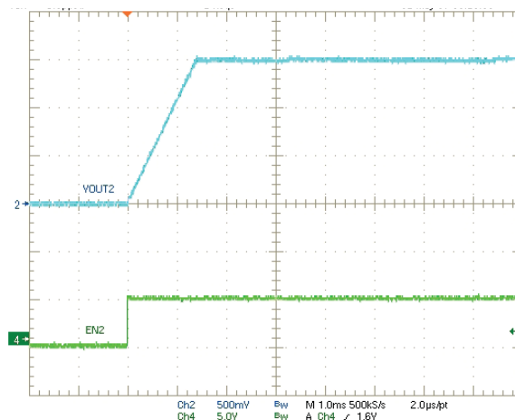
Startup VOUT2 1.5V
