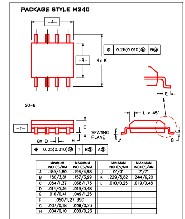
SO-8
